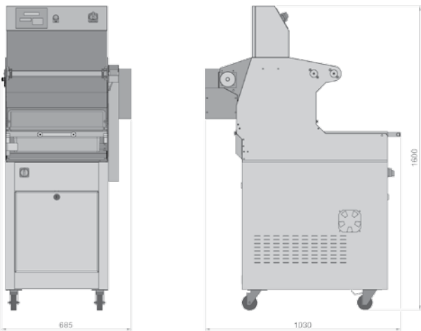
Lay-out ReeTray 25 VGM DIGIT
